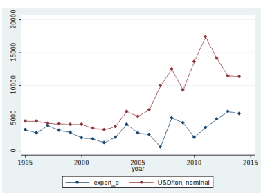
(j) Tin
