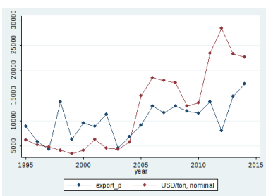
(k) Tungsten
