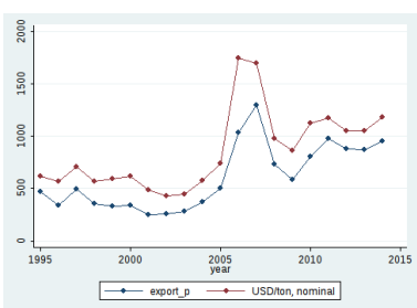
(l) Zinc
