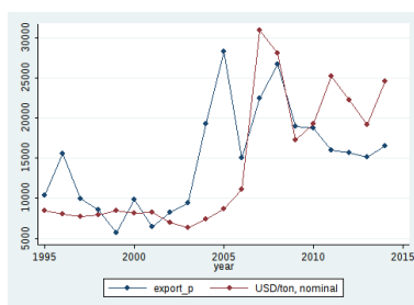
(b) Bismuth
