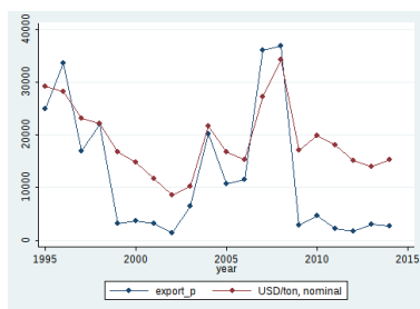
(d) Cobalt
